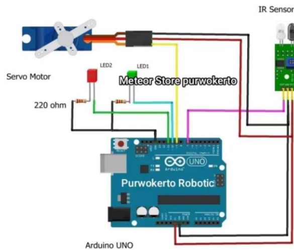
Gambar 6. Rangkaian Pintu Otomatis
